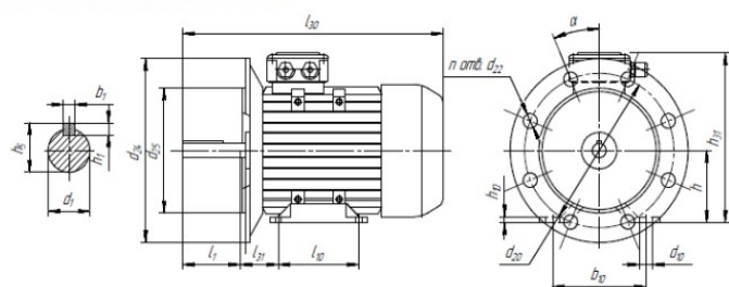
Присоединительные размеры**
